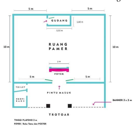
Gambar 10. Denah Gedung Pameran
